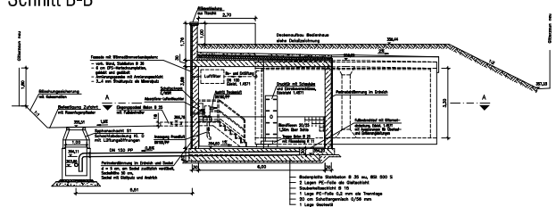
Schnitt B-B
