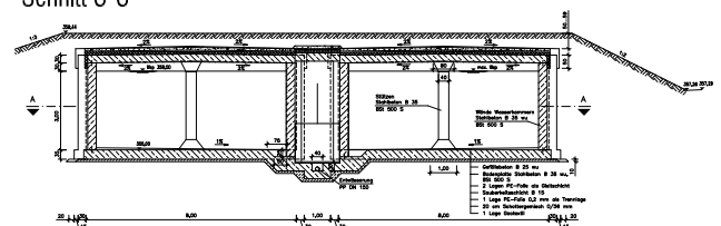
Schnitt C-C
