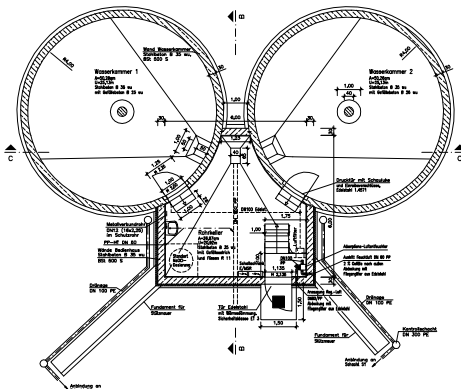
Planungsgrundriß Brillenbehälter
