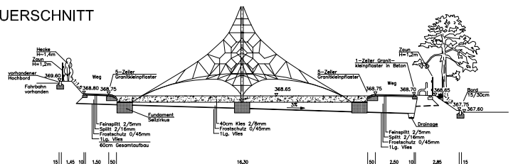
QUERSCHNITT
