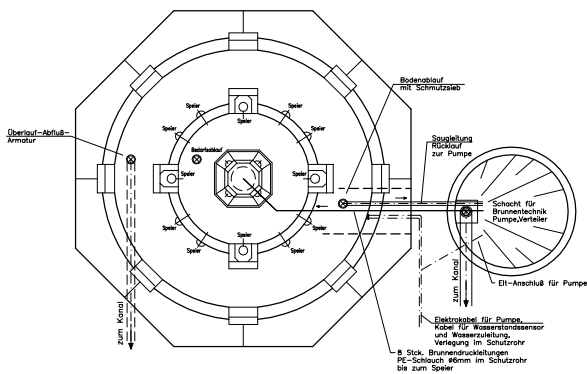
Draufsicht
